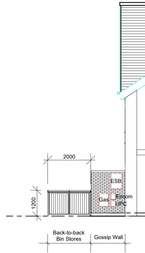
5 Type C Elevation 0483
