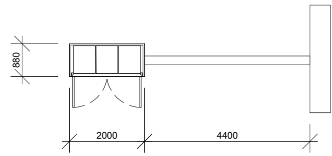
4 Type B Plan 0483
